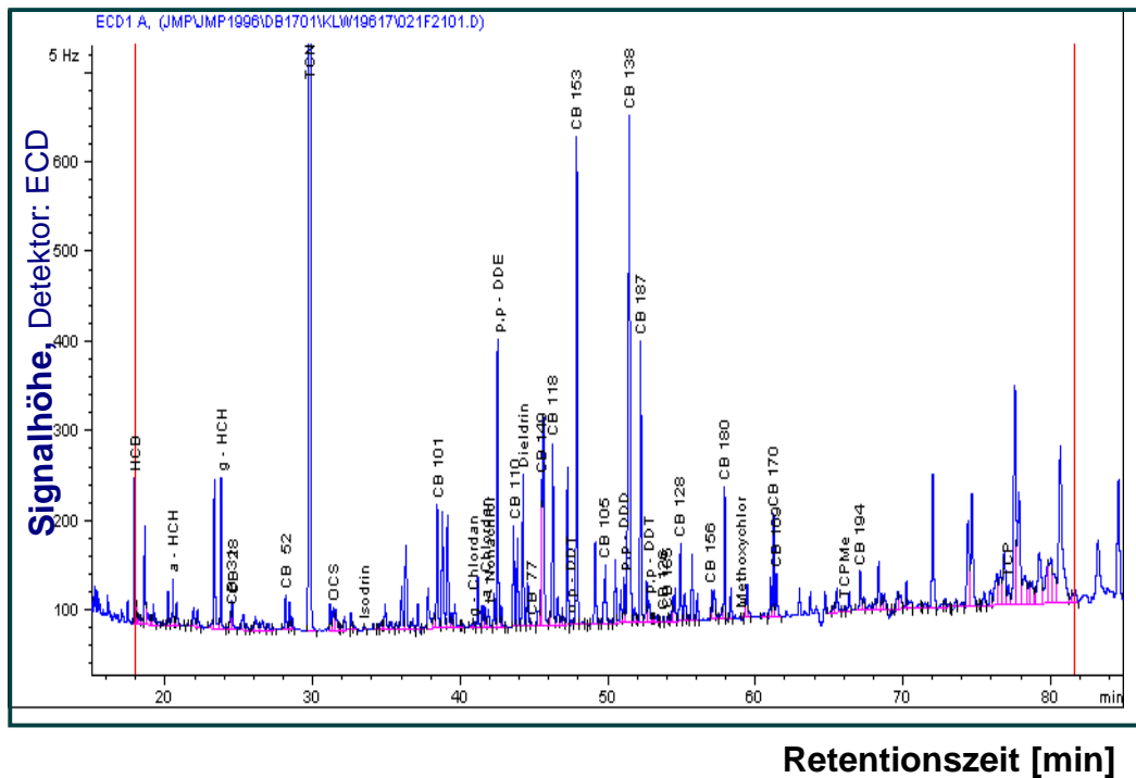
Abbildung 3: Spektrum einer Messung organischer Chlorkohlenwasserstoffe in einer Klieschenleber mit dem Gaschromatographen.
