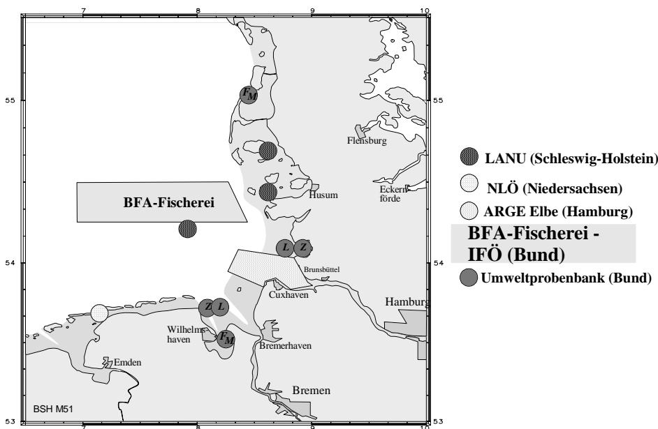
Abbildung 1: Probenahmegebiet der BFAFi und Stationen in der Deutschen Bucht für Schadstoffuntersuchungen in Organismen im Rahmen der nationalen (Gemeinsames Bund/Länder-Meßprogramm = BLMP) und internationalen (Joint Assessment and Monitoring Programme = JAMP) marinen Überwachungsprogramme
