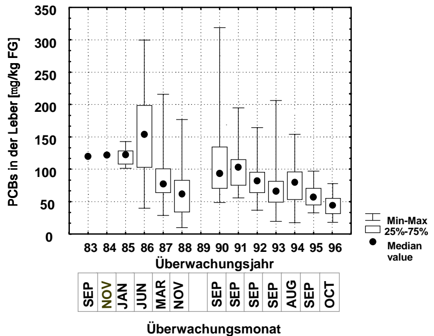
Abb. 5: Zeitliche Entwicklung der PCB-Konzentrationen (Summe von 7 PCBs: CB 28, 52, 101, 118, 138, 153 und 180) in Lebern (bezogen auf Frischgewicht (FG)) von Schollen aus der Deutschen Bucht 1983-1996
