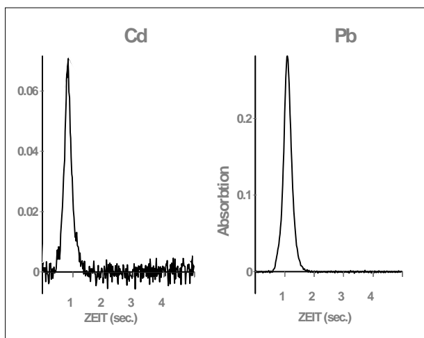
Abbildung 4: Spektren einer simultanen Messung von Cadmium und Blei in einer Dorschleber mit dem Atomabsorptionsspektrometer, (Man beachte den unterschiedlichen Maßstab für das Blei und Cadmiumsignal in Abb. 3 und 4.)
