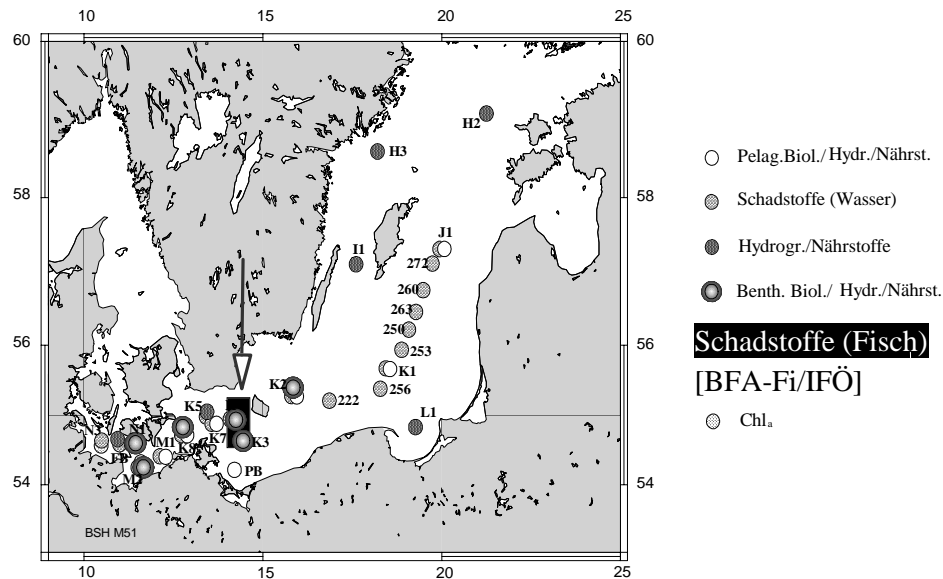
Abb.ildung 2: Probenahmegebiet der BFAFi und Stationen in der Ostsee für Schadstoffuntersuchungen im Rahmen der nationalen (Gemeinsames Bund/Länder-Meßprogramm = BLMP) und internationalen (Baltic Monitoring Programme = BMP/COMBINE) marinen Überwachungsprogramme
