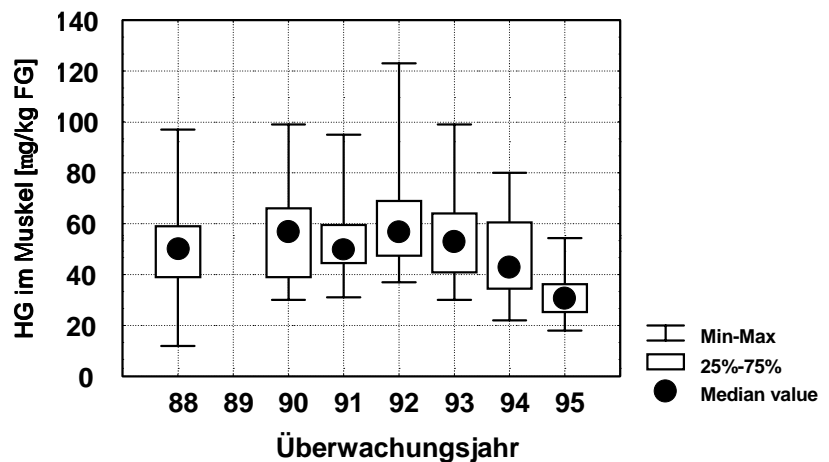
Abb. 6: Zeitliche Entwicklung der Quecksilberkonzentrationen im Muskelfleisch (bezogen auf Frischgewicht (FG)) von Schollen aus der Deutschen Bucht 1988-1995
