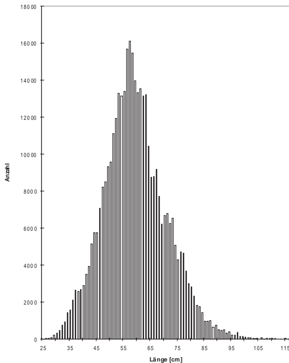
Abb. 7: Längenverteilung Kabeljau (Bäreninsel), ges. Fänge FMS „Kiel“, Mai-Juni 1997
