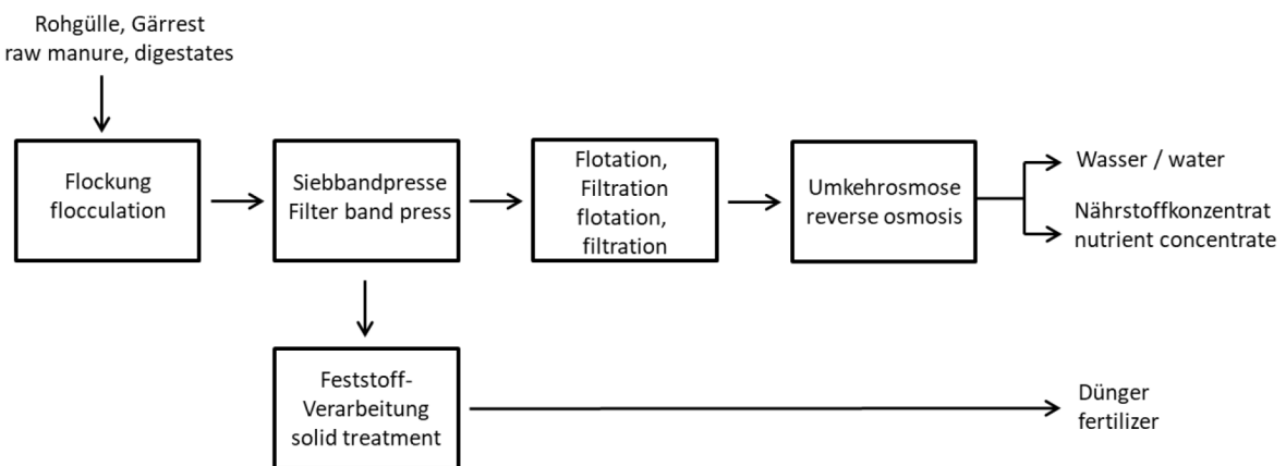
Bild 3: Schematische Darstellung des Gülleaufbereitungsverfahrens der WELTEC BIOPOWER GmbH Figure 3: Schematic flow diagram of the WELTEC BIOPOWER manure treatment process
